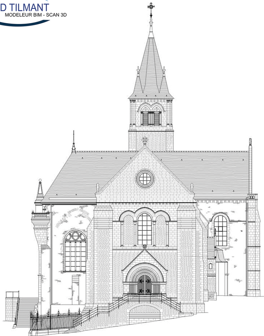
ÉLÉVATION OUEST - ÉTAT ACTUEL
